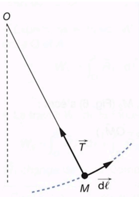
Pendule simple : la tension T ne travaille pas Figure 2
