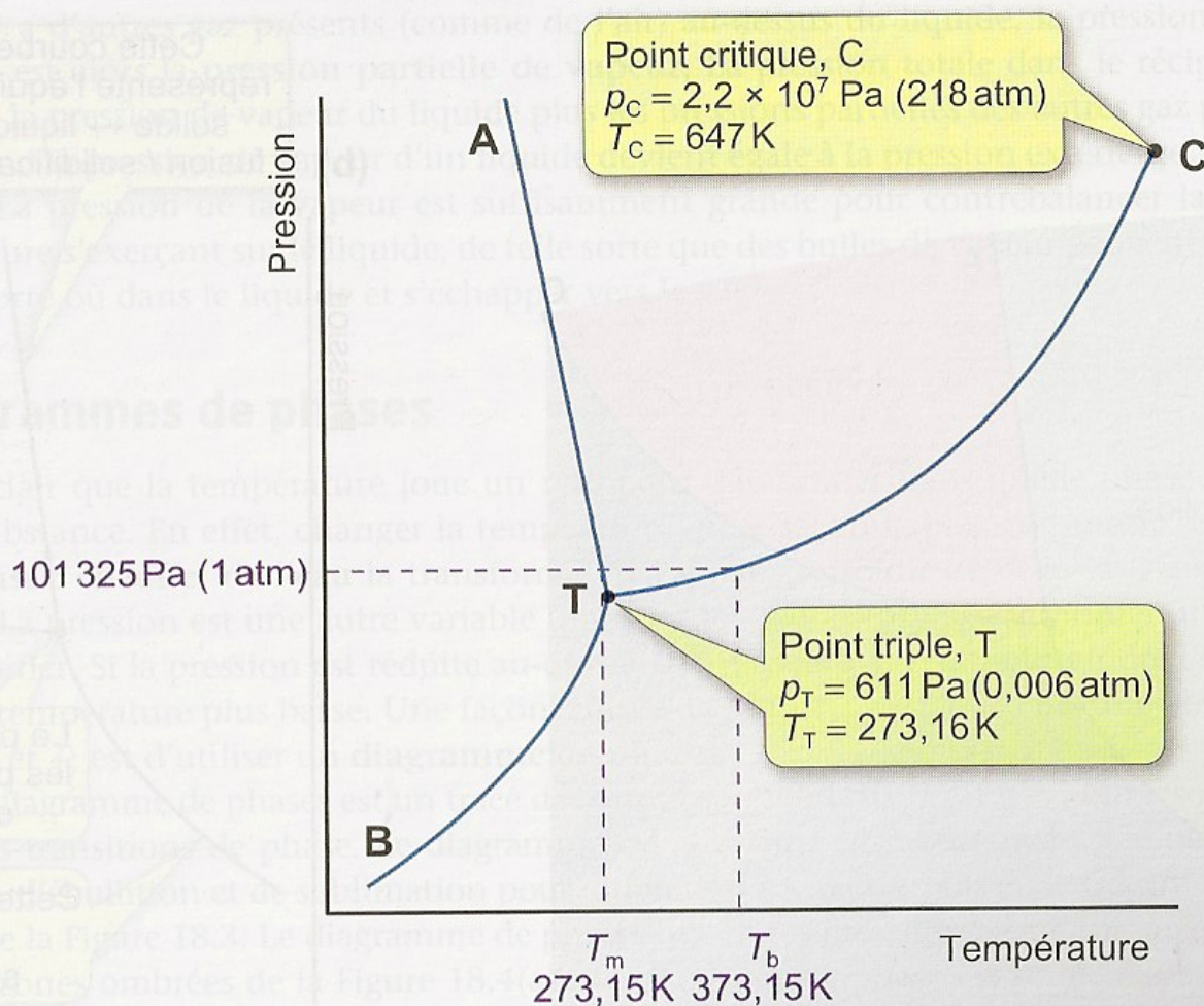
Figure 18.5 Diagramme de phases de l'eau (les diagrammes de phases ne sont en général pas tracés à l'échelle). La ligne horizontale pointillée violette, à 1 atm, coupe la ligne A–T de l'équilibre solide-liquide à la température normale de fusion de l'eau, et coupe la ligne C–T de l'équilibre liquide – vapeur à la température normale d'ébullition de l'eau.
