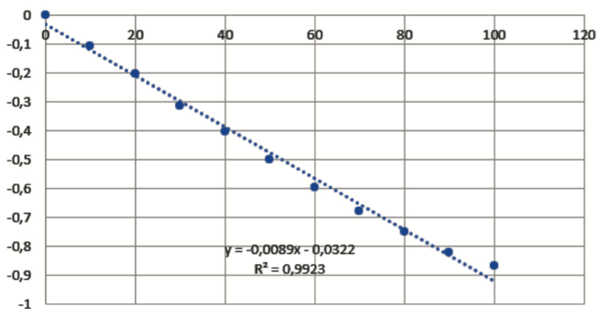
Graphe 3 : \frac{1}{0,01-2x} - 100 = f(t) 1/(0,01-2x)-100
